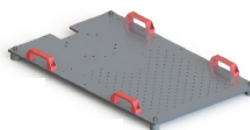
Basisplatte 800x500x10 mm Aluminium und 4 Plastikgriffe 180 Montagelöcher
